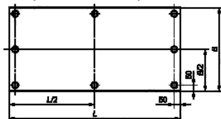
Схема расположения точек измерений толщины плит
